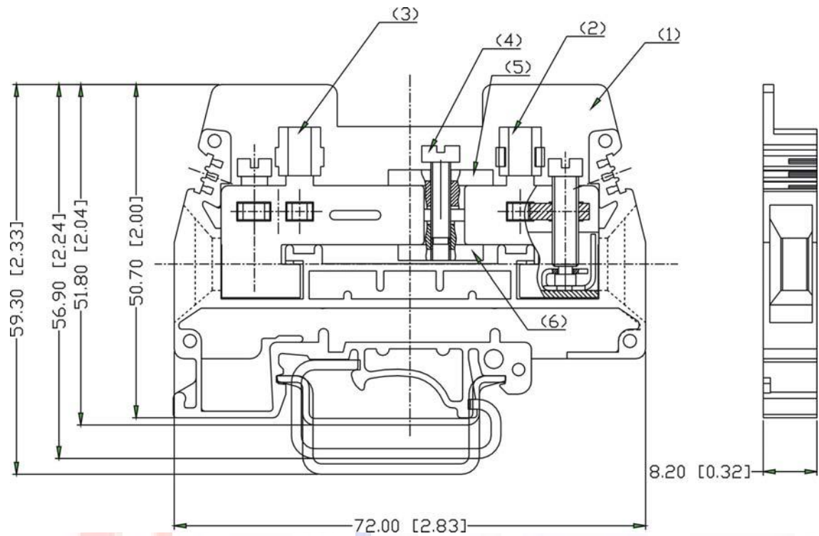
外形尺寸
